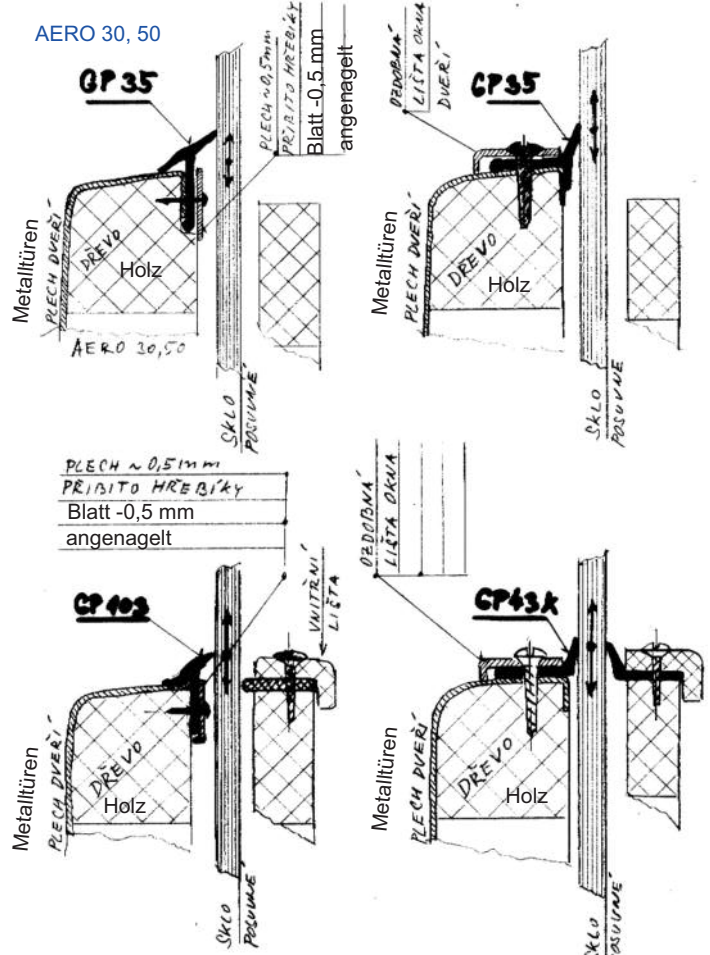
Příklady venkovního utěsnění spouštěcího okna,- Beispiele für Outdoor-Boot-Fenstern Abdichtung -
