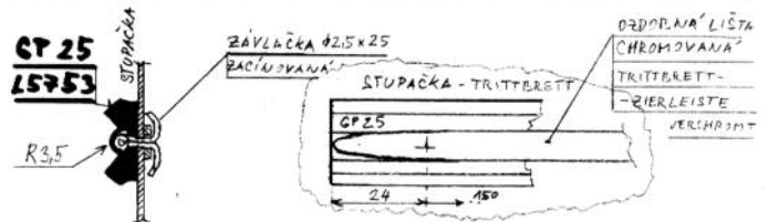
Uchycení gumy ozdobnou lištou ke stupačce vozů Aero 30, 50 - model 1939,-Packende Gummi Zierleisten Fußstütze bis Autos Aero 30, 50 - Modell 1939
