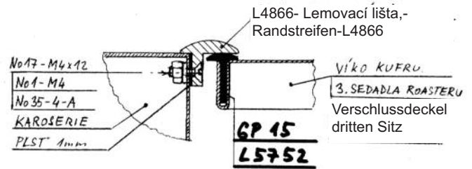
Utěsnění víka třetího sedadla karoserie - roaster Aero 30, 50 Verschlussdeckel dritten Sitz Körper - Röster Aero 30, 50
