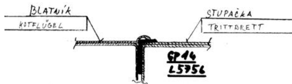
Umístění gumy mezi blatník a stupačku u vozů Aero 30, 50 - model 1939.- Lokalisierung von Gummi zwischen Kotflügel und Trittbrett des Aero 30 Autos, 50 Modell - die 1939. -
