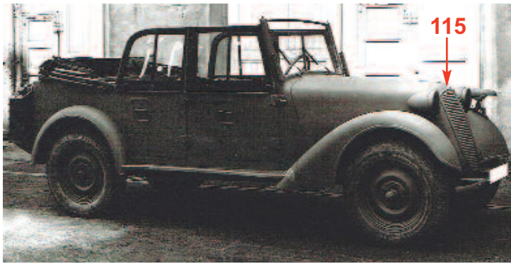
T57k - prototyp , ještě s blatníky T57b, na dalších již lem blatníku hladký. Vpředu tažné háky, užší stupačky než u T57b
