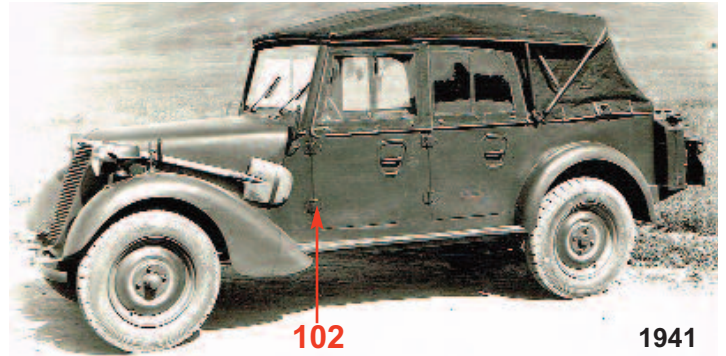
T57k - prototyp , ještě s blatníky T57b, na dalších již lem blatníku hladký. Vpředu tažné háky, užší stupačky než u T57b
