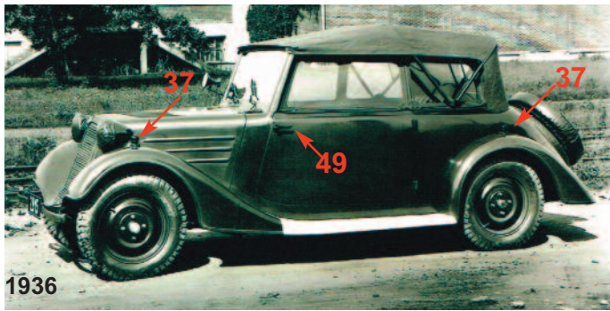
Sportovní vůz 4-místný - T57a - pro polici a armádu
