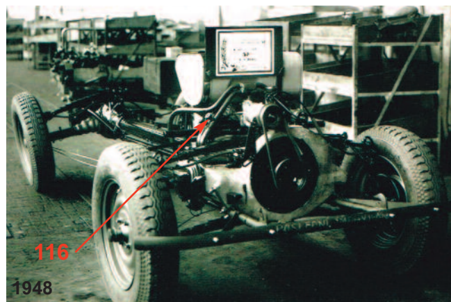
T57k - podvozek, použit i u posledních T57B
