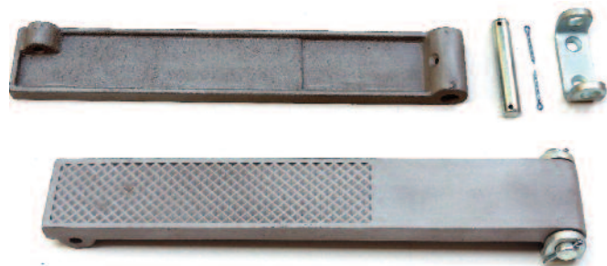
752306 Kč 2360,- Pedál plynu - odlitek , - Gaspedal 752309 Kč 330,- Ložisko pedálu plynu , - Lager des Gaspedals 752311 Kč 225,- Čep , - Bolcen 752306-K Kč 2810,- Pedál plynu -kompletní , - Gaspedal- komplett
