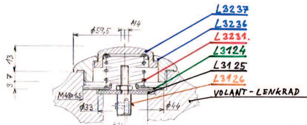
Sestava klaksonu,-
