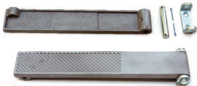
752306 Kč 2450,- Pedál plynu - odlitek , - Gaspedal 752309 Kč 335,- Ložisko pedálu plynu , - Lager des Gaspedals 752311 Kč 225,- Čep , - Bolcen 752306-K Kč 2980,- Pedál plynu -kompletní , - Gaspedal- komplett
