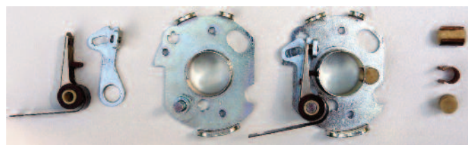
K-Scintila 605 Kč,- Kontakty zapalování SCINTILA,- Unterbrecherkontakt Scintila (Aero 30,50, Tatra 57,75,87)
