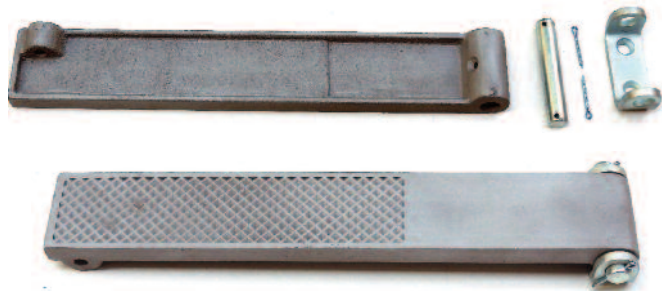
752306 Kč 2995,- Pedál plynu - odlitek , - Gaspedal 752309 Kč 405,- Ložisko pedálu plynu , - Lager des Gaspedals 752311 Kč 260,- Čep , - Bolcen 752306-K Kč 3495,- Pedál plynu -kompletní , - Gaspedal- komplett
