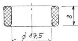
G- T600.05.61 95,-Kč Těsnící kroužek dolní (8 ks na vozidle)
