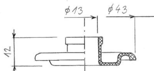
G- T600.09.06 170,-Kč Těsnící kroužek nástrčky kabelu (zabraňuje úniku chladícího vzduchu kolem zapalovacích svíček) (4 ks na vozidle)
