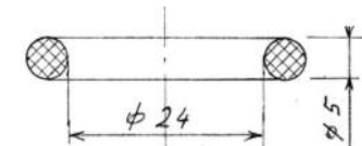
G- T600.05.37 80,-Kč Těsnící kroužek horní (8 ks na vozidle)
