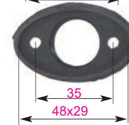
G-KL- 1 Náhradní pryž.podl. Ersatz Gummi- Unterlegscheibe
