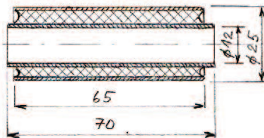
G-600.44.04 Kč 610,- Pouzdro předního pera,- Büchse-gummi (při náhradě bronzového pouzdra se zkracovalo o 2 mm - viz. díl.příručka) (4 ks na vozidle)
