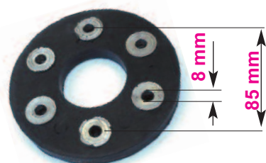
A 1129 Kotouč hardy spojky ,-Hard-Kupplungsscheibe L38 Kotouč hardy spojky do 1600 vozu,- Hardy-Kupplungsscheibe 120/48x14,5 mm Aero 500,662,1000,30
