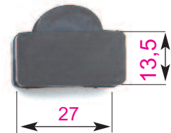
G -KD -3 Gumové vodítko dveří,- Gummi Tür Keil
