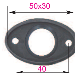
G-KL- T - 1 Náhradní pryž.podl. šikmá pro vyrovnání sklonu dveří,- Ersatz Gummi-Unterlegscheibe- Leaning Tür zu entzerren sklon 8 stupňů,-Steigung 8 Grad
