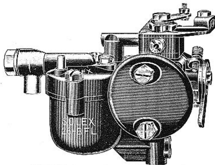
Abb. 2. BFH-Vergaser mit automatischer Startvorrichtung Horizontale Anordnung
